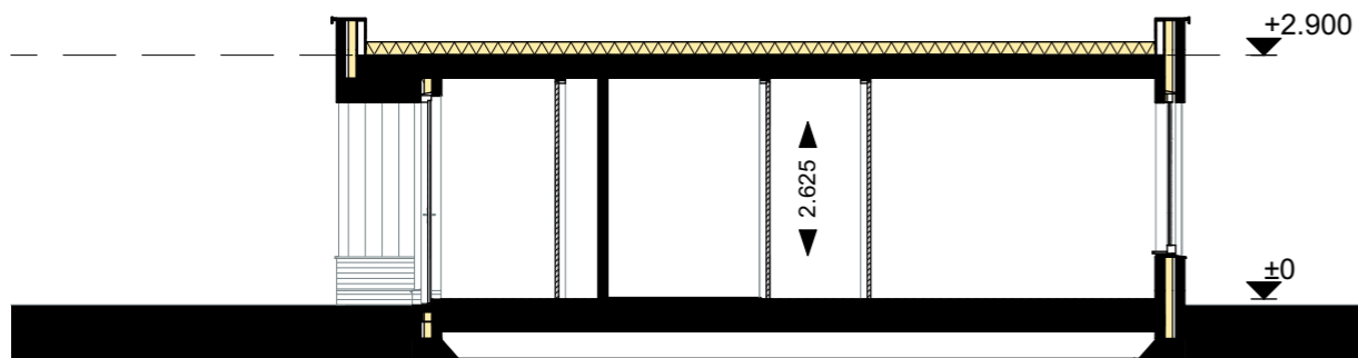
Doorsnede
